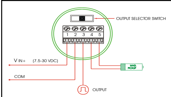
Model PET-4 TTL/CMOS (0-5 VDC)
